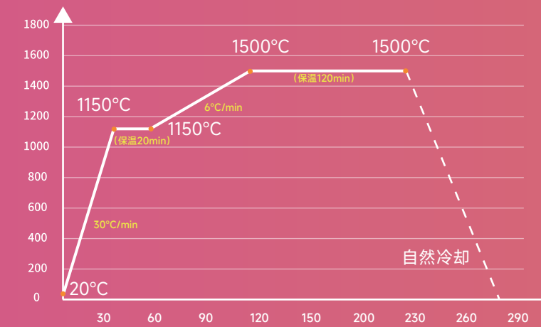
快烧3D多层六单位以内缺失位完全烧结曲线
