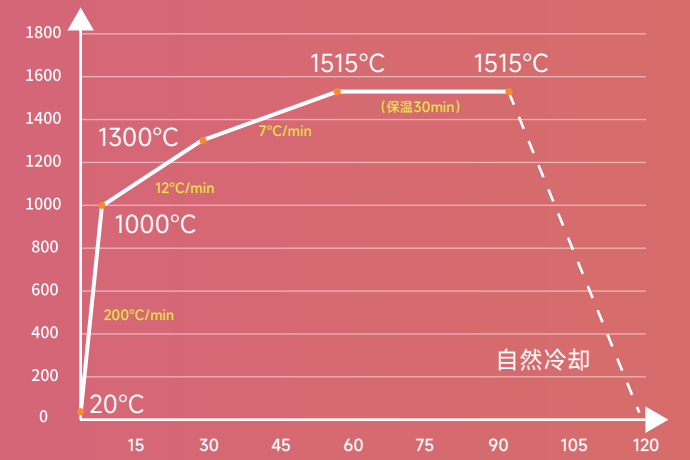
快烧3D多层三单位以内缺失位完全烧结曲线
