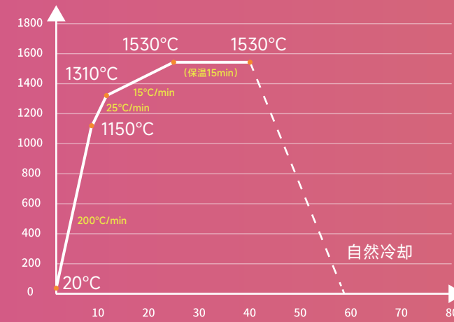
快烧3D多层单颗不含缺失位完全烧结曲线
